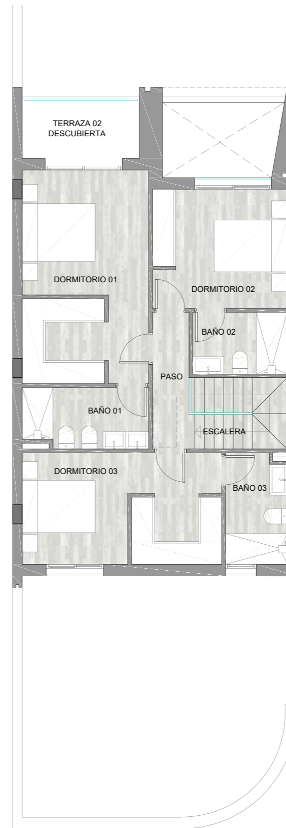
PLANTA PRIMERA
