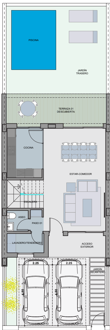
PLANTA BAJA.
