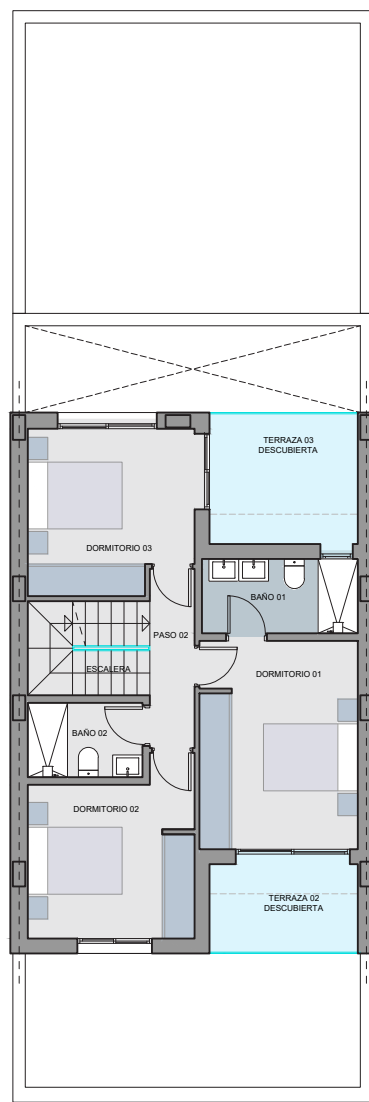
PLANTA PRIMERA.
