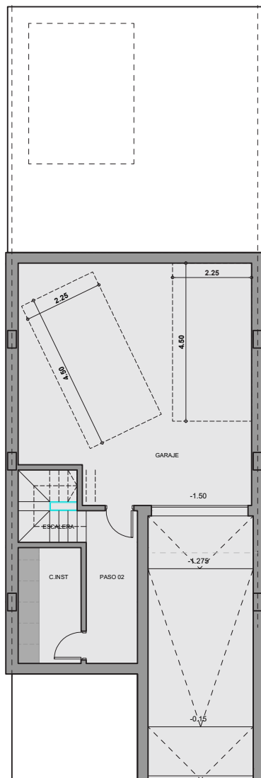
PLANTA SÓTANO
